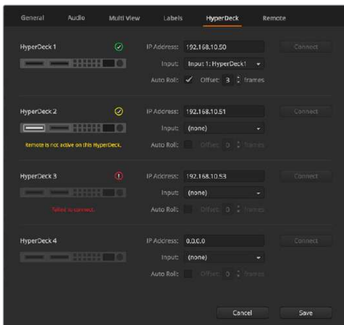
Подключение рекордеров HyperDeck
